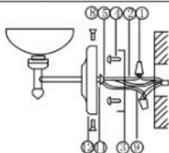
Bild 3 Wandleuchte
