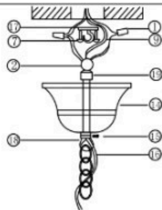
Bild 2 Pendelleuchte
