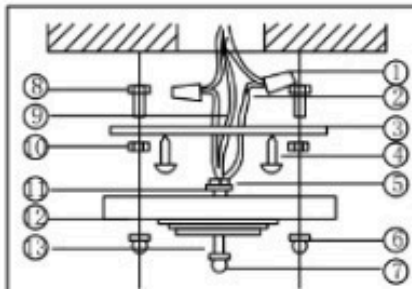
Bild 1 Deckenleuchte
